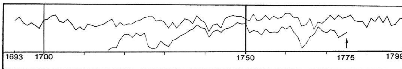
Figur 3. Referansekurve av gran for perioden 1693 til 1799, og den daterte årringkurven med siste årring fra 1775 innpasset nederst.
